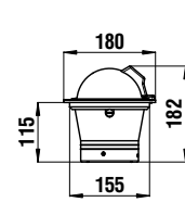
Bussola magnetica installazione a inc. orizzontale Horizontal flush mounted magnetic compass
